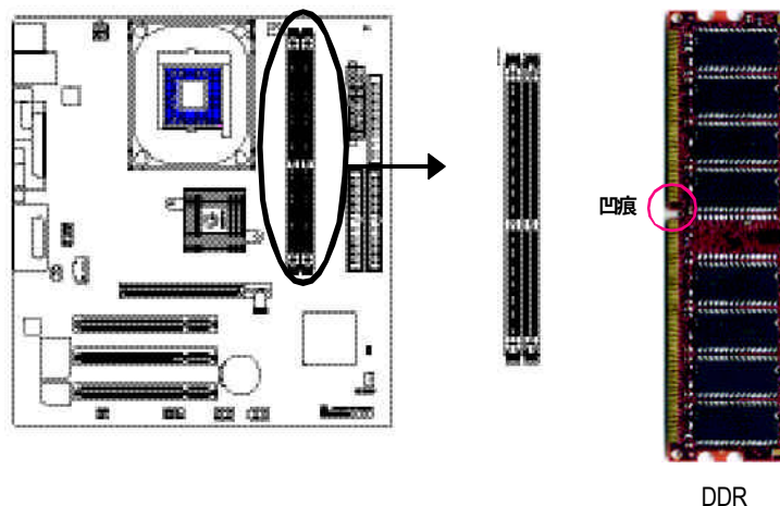
使用 Unbuffered DDR DIMM 時的總記憶容量
