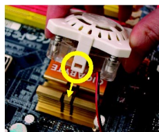
図 1 Cool-Plus をヒートシンクにインストールするには、下記のようにヒートシンクの溝に沿い、両側に向け拡張部を位置合わせしてください。正しい位置に填まるまで、しっかりと押し込んでください。
