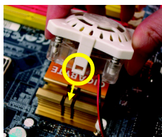
圖 1. Cool-Plus 的安裝是有方向性的，須將 Cool-Plus 的二端扣環對齊北橋散熱片的勾點，再施力將 Cool-Plus 下壓至扣住。
