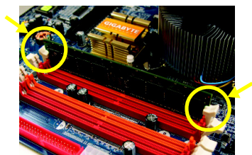
圖 2. 一旦確實壓入插槽內，兩旁的卡榫便會自動向內卡住記憶體模組予以固定。試著輕輕搖動記憶體模組，若不搖晃則表示安裝完成。
