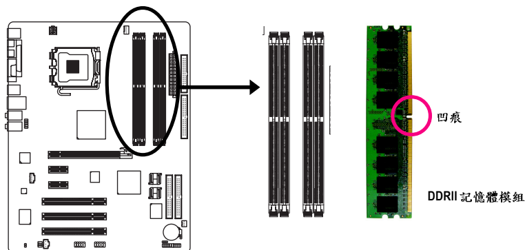
圖 1. 記憶體模組有一個凹痕，所以只能以一個方向插入。請扳開記憶體模組插槽卡榫，以雙手按在記憶體模組上邊兩側，以垂直向下平均施力的方式，將記憶體模組下壓推入插槽。
