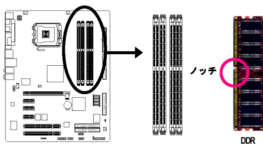
図 1 DIMM ソケットにはノッチがあり、DIMM メモリモジュールは一方向のみに挿入するようになっています。DIMM メモリモジュールを DIMM ソケットに垂直に挿入し、押し下げてください。
