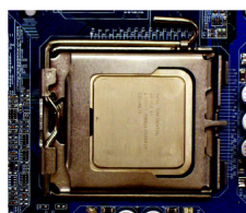
Fig. 4 Une fois que le processeur est installé correctement, remplacez le couvercle en plastique et poussez le levier métallique dans sa position originale.
