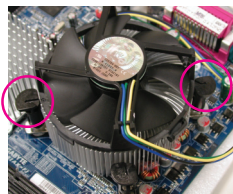
Рис. 3 Разместите теплоотвод на процессоре. Убедитесь, что крепежные штырьки расположены над отверстиями в системной плате. Нажмите на головки штырьков, одновременно поворачивая их в направлении, противоположном стрелке.
