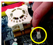
圖 2. Cool-Plus 固定住後，再將電源線接至主機板上的 NB_FAN 插座即完成。
