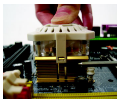
圖 3. 若要拆下 Cool-Plus 時，請先拔除電源線，再將 Cool-Plus 向下壓，以一字螺絲起子將 Cool-Plus 的扣環向外扳開即可。
