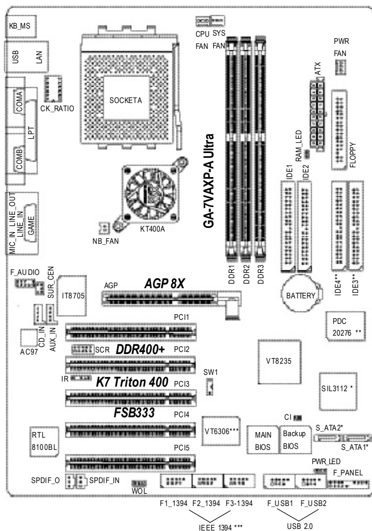
KT400A 系列主機板 Layout 圖
