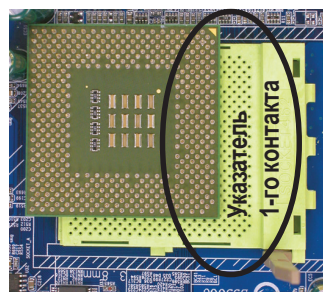
Процессор (вид снизу)
