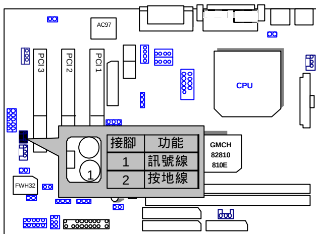
JP14 : 偵測外殼開啟功能
