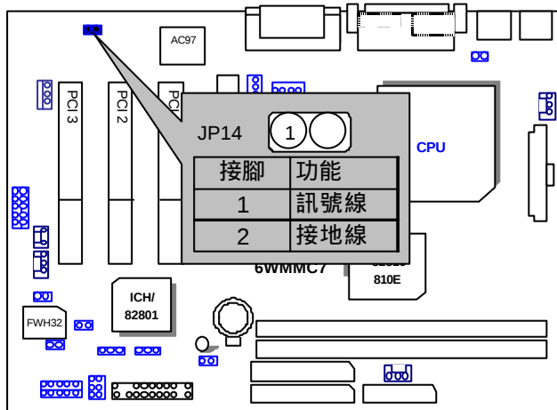
JP14 : 偵測外殼開啟功能
