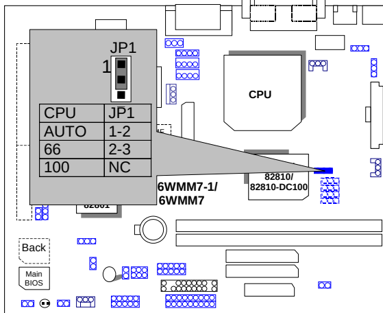
圖 1: other chipset CPU速度設定
