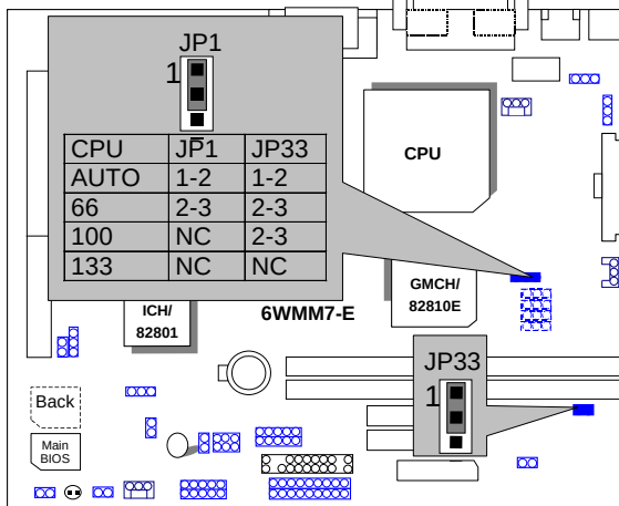
圖 2: 82810E chipset CPU 速度設定
