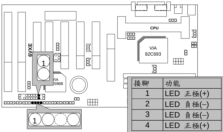
IR : 紅外線連接端 (Infrared Connector) (Optional)
