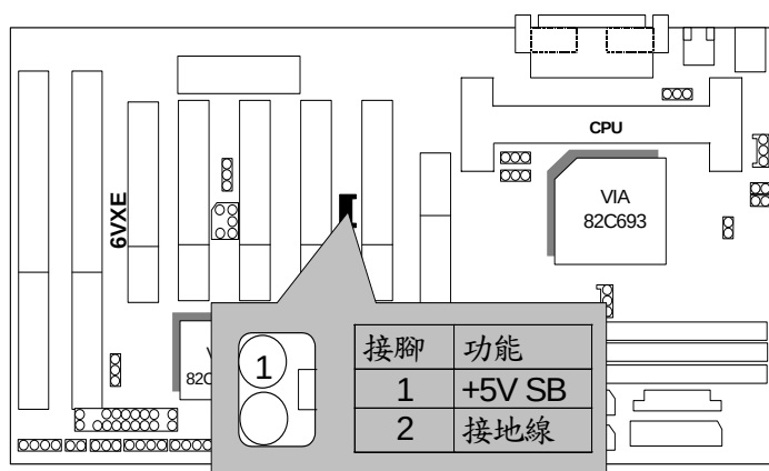
J16:內接型數據機開機功能
