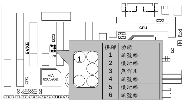
JP8 SB-LINK : PCI 音效卡支援接頭
