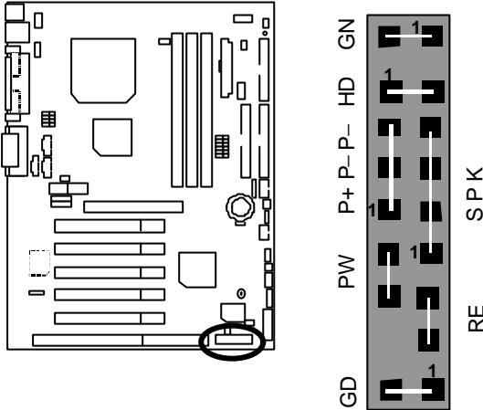
J2: 2x11 Pins 接腳說明
