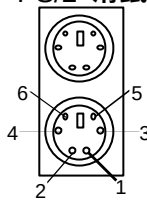
PS/2 鍵盤
