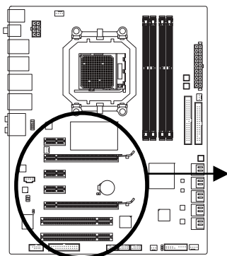
PCI Express x1 插槽
