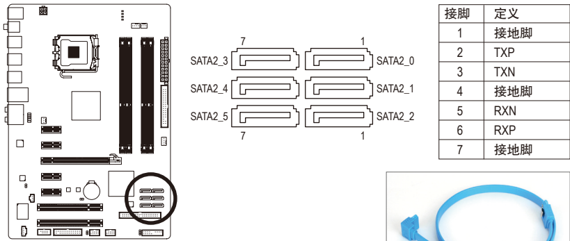
请将SATA排线的L型接头连接至SATA硬盘。
