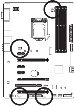
SYS_FAN1/SYS_FAN2/SYS_FAN3
