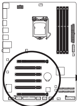
PCI Express x16 スロット
