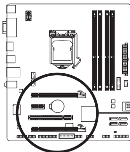
PCI Express x16 スロット (PCIEX16)
