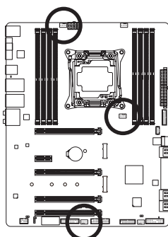
SYS_FAN1
