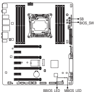
BIOS LEDインジケータ:
