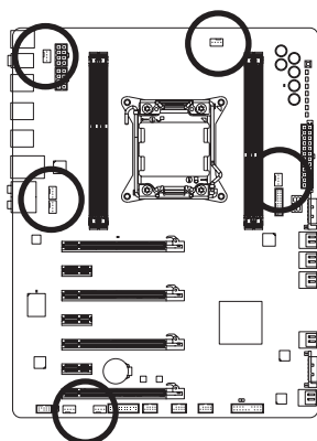
FAN1/FAN2/FAN5/FAN6
