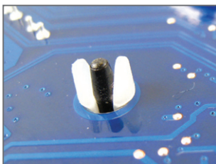
Fase 5: Dopo l'installazione, controllare la parte posteriore della scheda madre. Se i perni sono inseriti come mostrato nella precedente immagine, l'installazione è completata.
