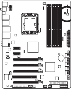
PW_SW: Stromschalter RST_SW: Rücksetzschalter
