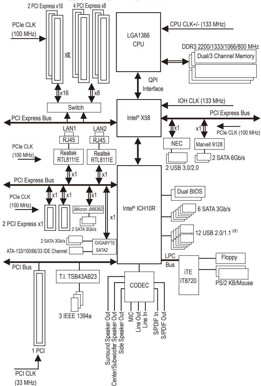
GA-X58A-UD5主板芯片组功能框图
