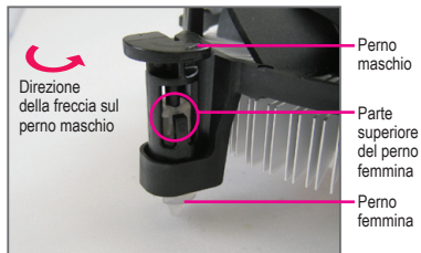
Fase 2: Prima di installare il dissipatore, notare la direzione freccia sul perno maschio. (Girando il perno nella direzione indicata dalla freccia si rimuove il dissipatore, girando in senso inverso si installa il dissipatore.)
