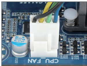
Fase 6: Infine, collegare il connettore d'alimentazione del dissipatore di calore CPU al connettore ventolina CPU (CPU_FAN) della scheda madre.
