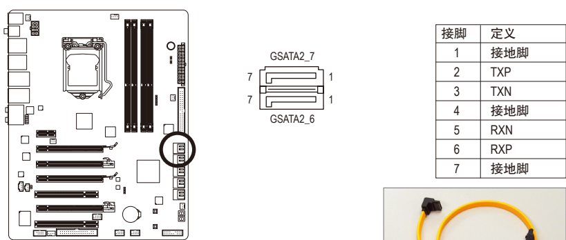
请将SATA 3Gb/s排线的L型接头连接至SATA硬盘。
