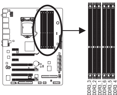
► Tableau des configurations de la mémoire à canal double
