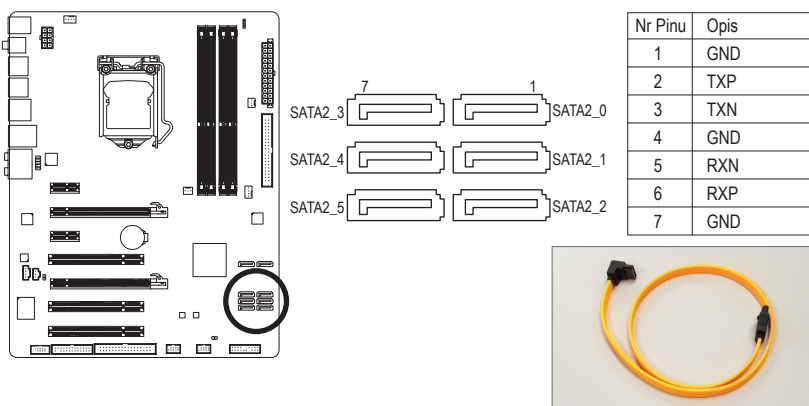
Końcówkę kabla SATA 3Gb/s (w kształcie litery L) podłącz do dysku twardego SATA.
