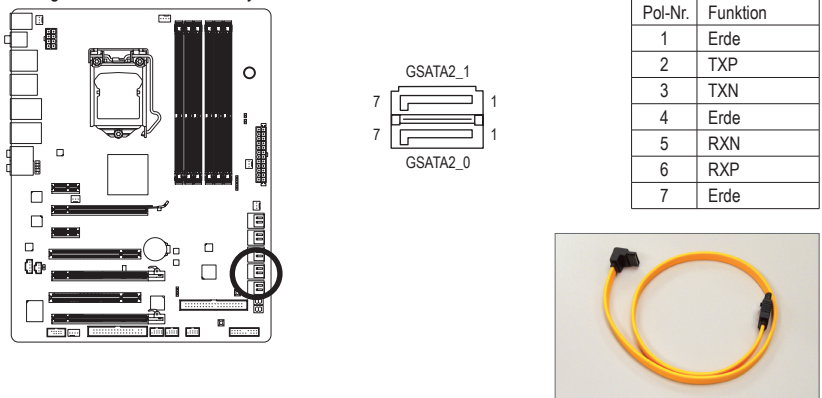
Bitte verbinden Sie das L-förmige Endes des SATA 3Gb/s-Kabels mit Ihrer SATA-Festplatte.
