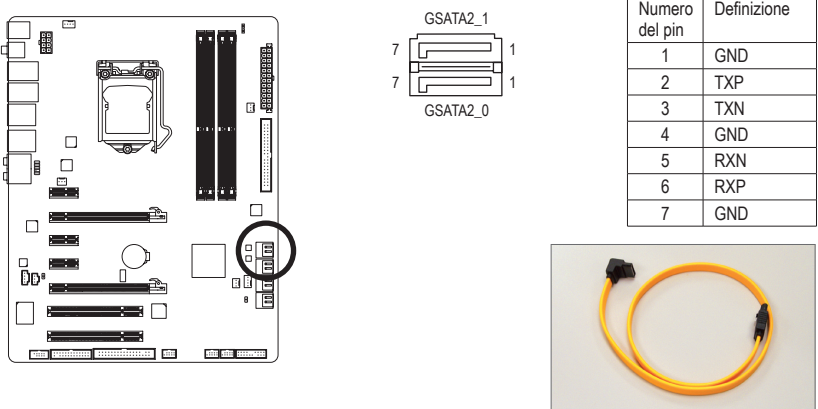
Collegare il terminale a forma di L del cavo SATA 3Gb/s al disco rigido SATA.
