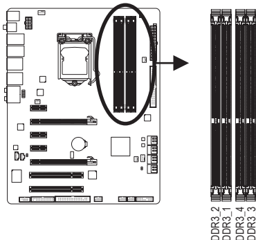
» Dual Channel-Speicherkonfigurationstabelle
