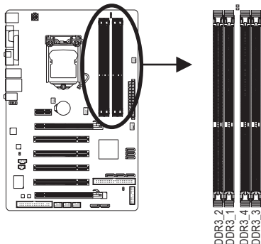
►► Dual Channel Speicherkonfigurationstabelle
