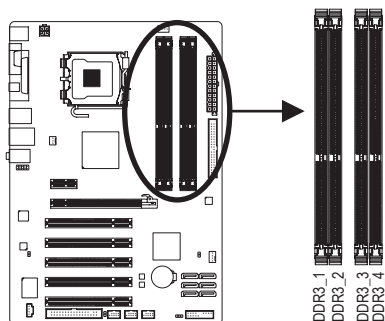
► Tabella di configurazione memoria Dual Channel
