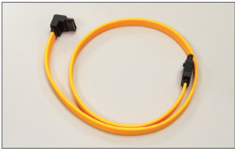
Collegare il terminale a forma di L del cavo SATA 3Gb/s al disco rigido SATA.
