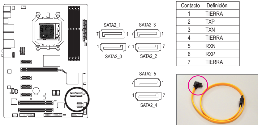
Conecte el extremo con forma de L del cable SATA de 3 Gb/s a la unidad de disco duro SATA.
