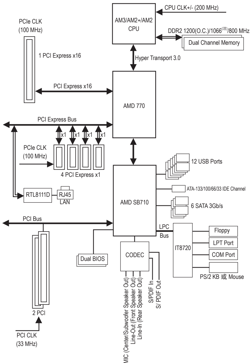
GA-MA770-ES3主机板功能方块图
