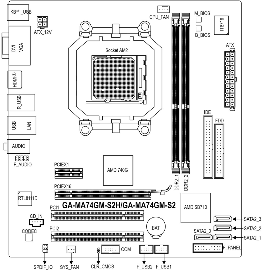
GA-MA74GM-S2H/GA-MA74GM-S2 主板配置图
