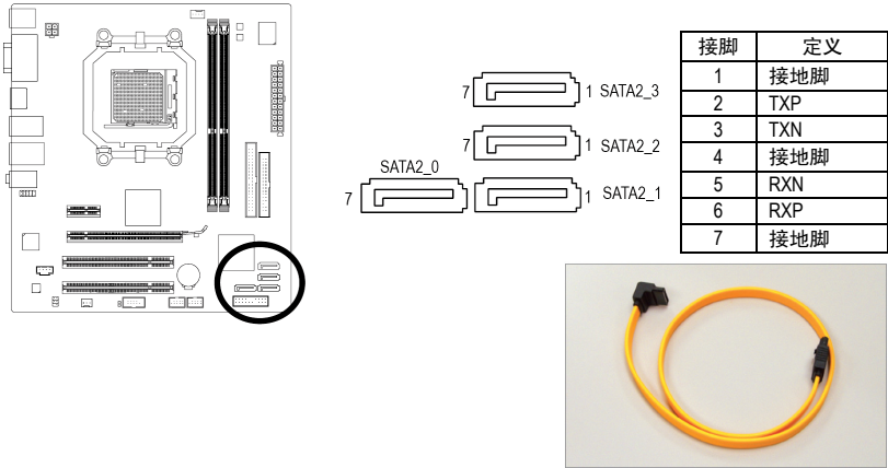
请将 SATA 3Gb/s 排线的 L 型接头连接至 SATA 硬盘。
