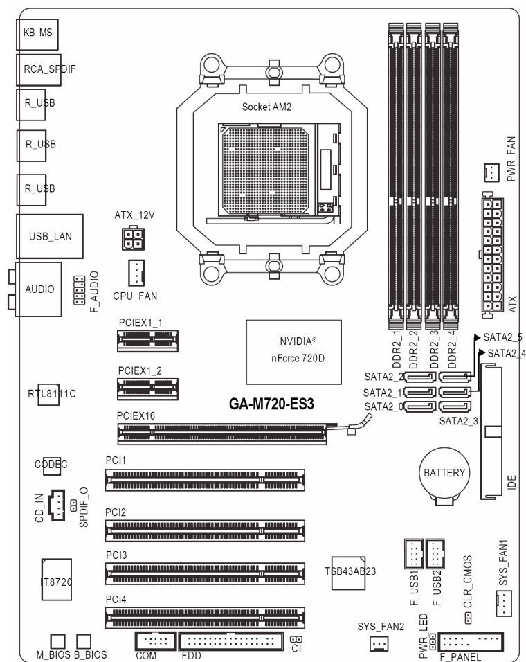
GA-M720-ES3 主板配置图
