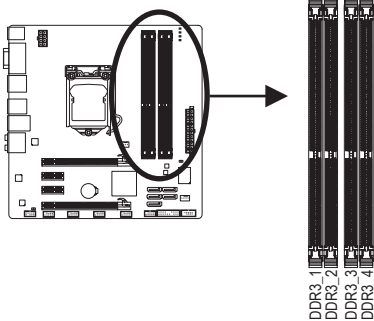
▶ 듀얼 채널 메모리 구성표
