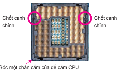
Đế cắm CPU LGA1156
