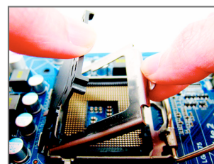
مرحله سوم: قاب نگه دارنده فلزی بر روی سوکت پردازنده را از جای خود بلند کنید. (برای محافظت از سوکت پردازنده، همیشه پوشش محافظ سوکت را مواقعی که پردازنده روی سیستم نصب نیست در جای خود قرار دهید.)
