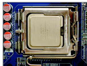
مرحله پنجم: هنگامی که پردازنده به درستی در جای خود قرار گرفت، قاب نگه دارنده را به جای خود بازگردانده و آن را به وسیله پایین آوردن اهرم قفل کنید.
