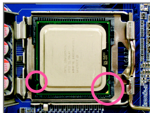
مرحله چهارم: پردازنده را میان انگشتان شصت و اشاره خود نگه دارید. پین شماره یک پردازنده را ببابید (با توجه به مثلث طلایی رنگ) و آن را با پین شماره یک بر روی سوکت پردازنده هم جهت کنید. (همچنین می توانید با استفاده از فرورفتگی های بر روی پردازنده و برآمدگی های بر روی سوکت، جهت صحیح قرار گیری آن را پیدا کنید.)
