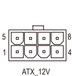
ATX_12V:
