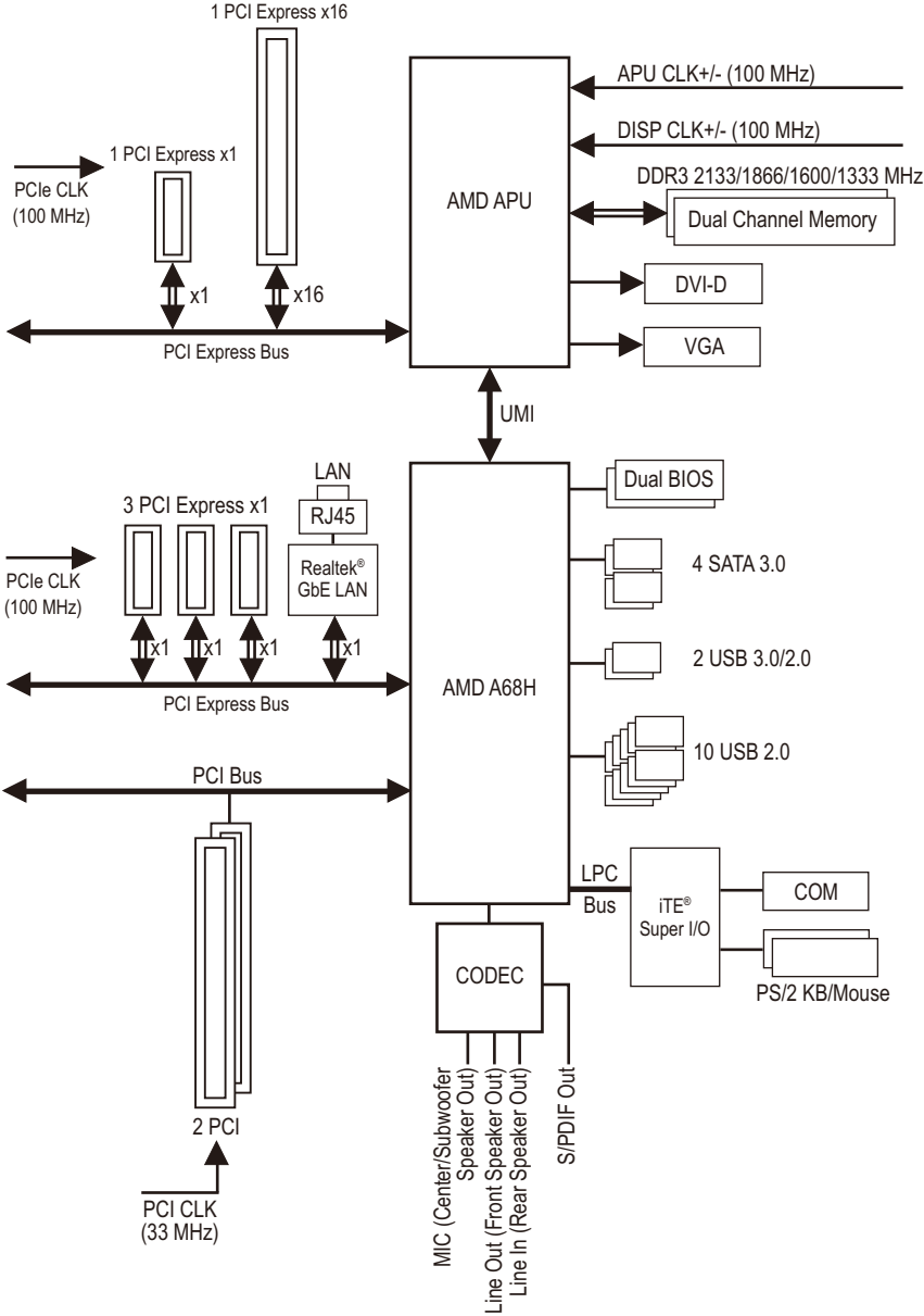
GA-F2A68H-DS3主板功能框图
