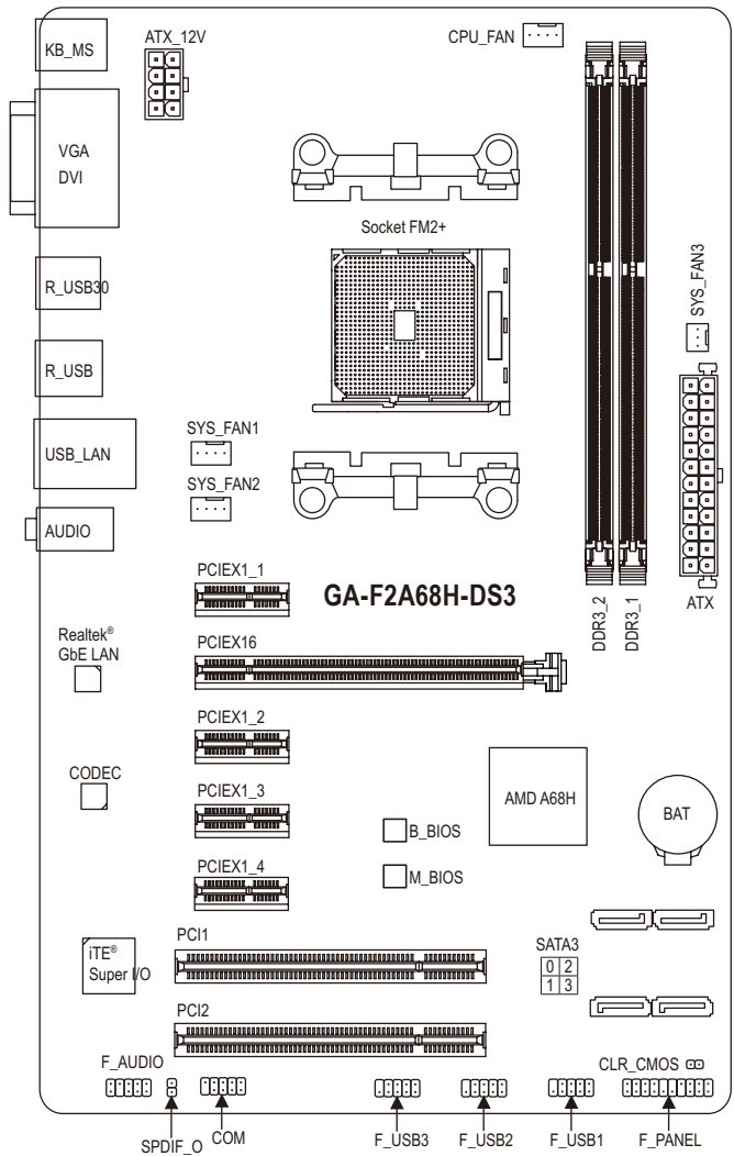
GA-F2A68H-DS3主板配置图
