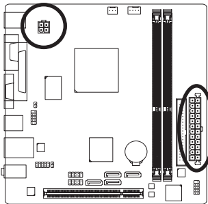
ATX:
