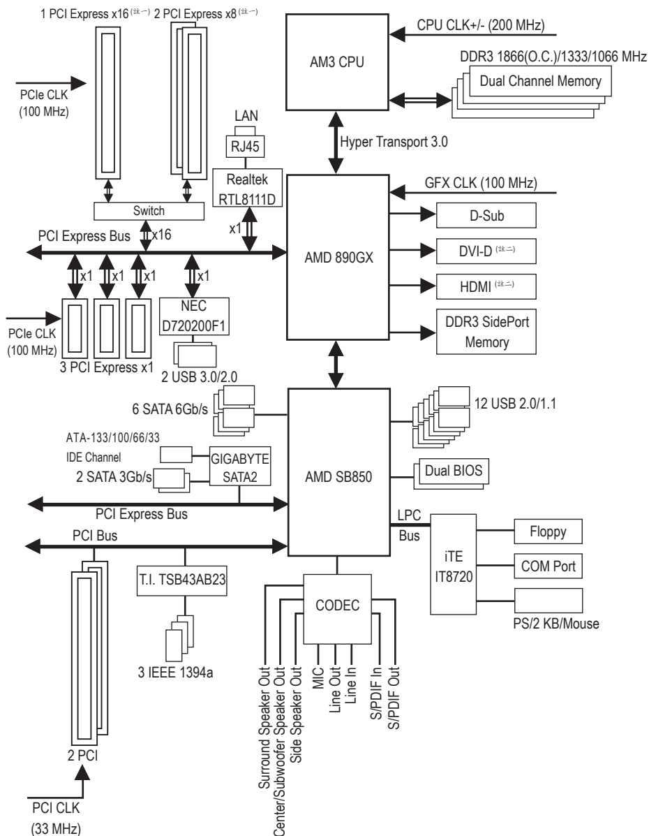
GA-890GPA-UD3H主機板功能方塊圖
